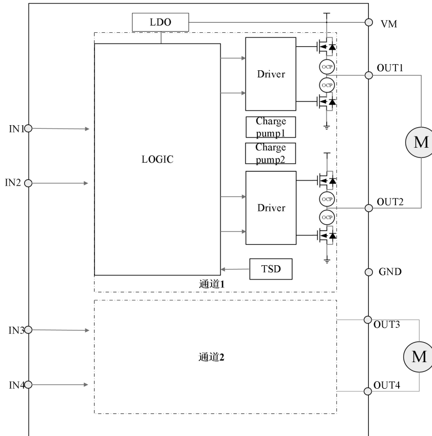
图 1 : GC3909 内部框图
