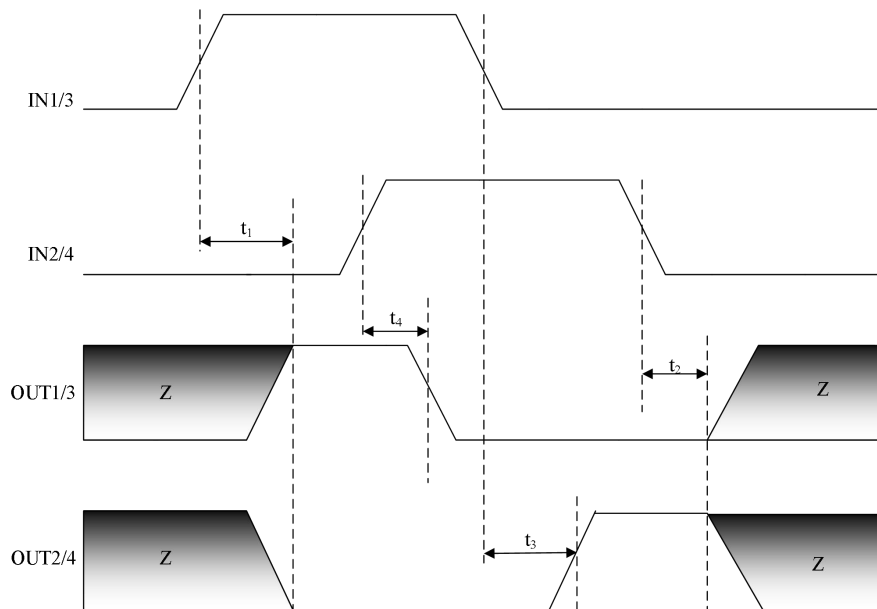
图2 GC3909 输入输出时间参数 1
